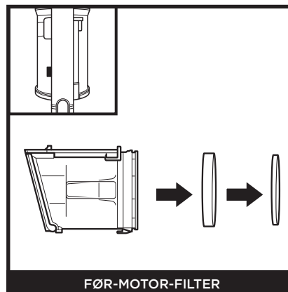
FØR-MOTOR-FILTER
