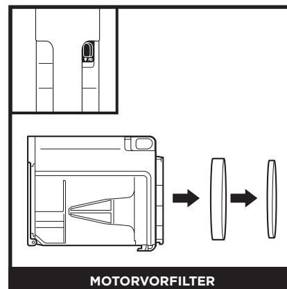
MOTORVORFILTER
