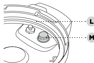
Onderkant drukdeksel
